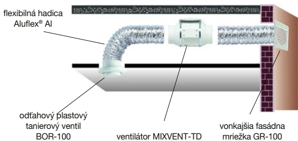
priklad inštalácie MIXVENT-TD KIT
